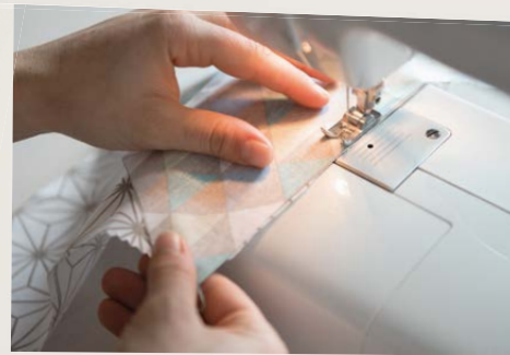
2. Alle Seiten, wie abgebildet, mit 1-cm-Nahtzugabe absteppen.
